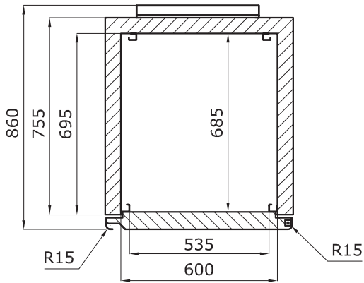
A-A
